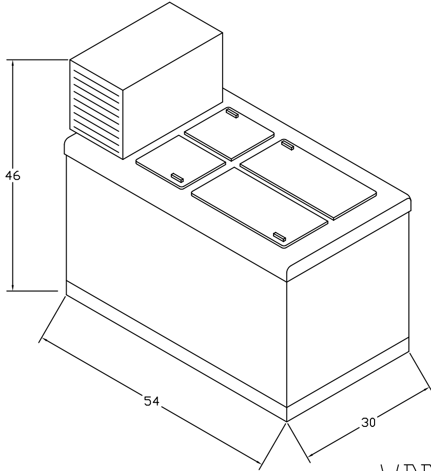
VBD-8 MOTOR TOP
